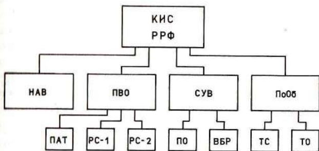
КИС-РРФ: хијерархијски дистрибуирани командно-информациони систем речног артиљеријско-ракетног брода
