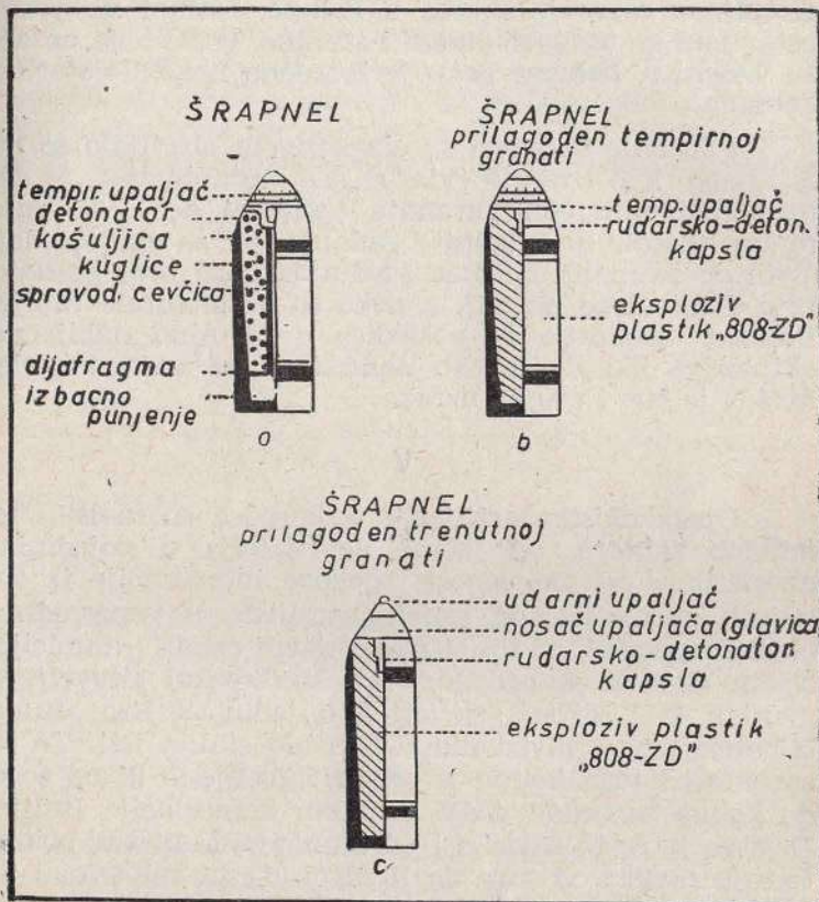
Skica 7. — »Adaptacija« šrapnel-granate
