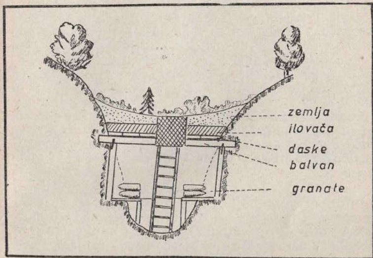
Skica 9. — Sklonište za art. municiju
