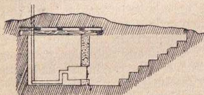
Profil zemljanke
